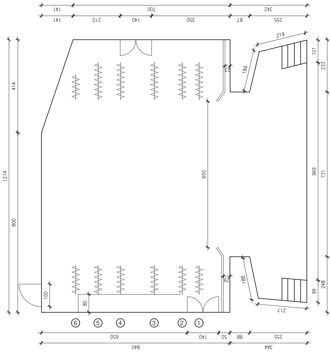
TLOCRT POZORNICE M 1:100
